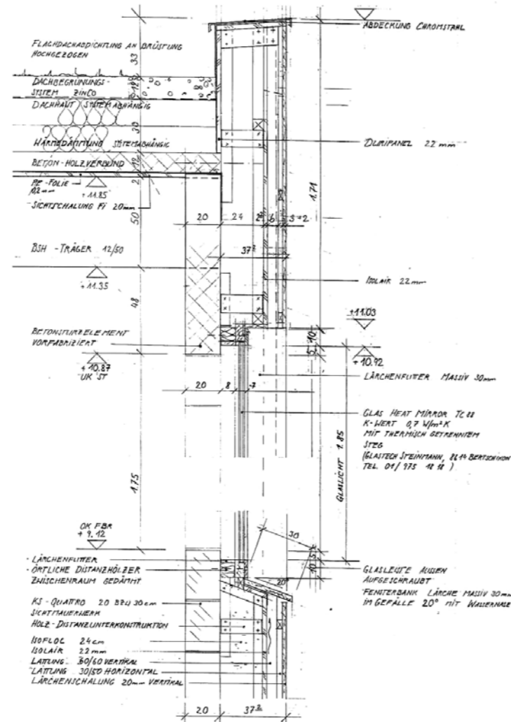
Detailschnitt West- und Ostfassade: einfache Verbindungen der Baustoffe, die leicht voneinander getrennt werden können.
